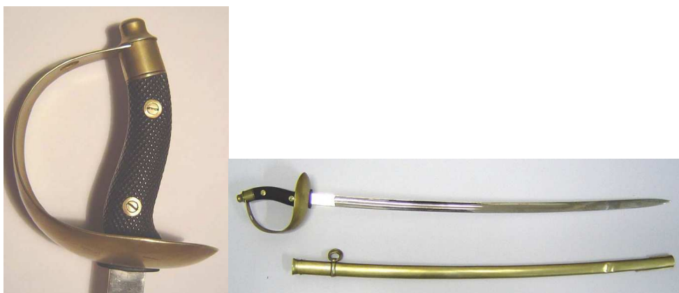
SABLE “MODELO ROBERT”. CAZOLETA SIN EMBLEMA, VAINA Y PIEZAS METÁLICAS DE LA EMPUÑADURA CON BAÑO AMARILLO (¿?). HOJA (784 x 23 mm flecha 23 mm), INSCRITA “Fca DE TOLEDO 1897”. Fotos Eduardo Gorostiza
