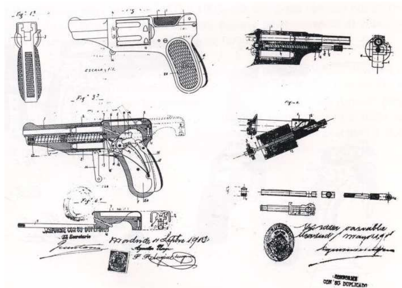
DISEÑOS DEL REVOLVER AUTOMÁTICO DE BOLSILLO, PATENTADO POR TORIBIO ZULAICA EN 1906
