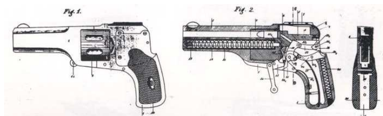
DISEÑOS DEL REVOLVER AUTOMÁTICO DE BOLSILLO, PATENTADO POR TORIBIO ZULAICA EN 1904
