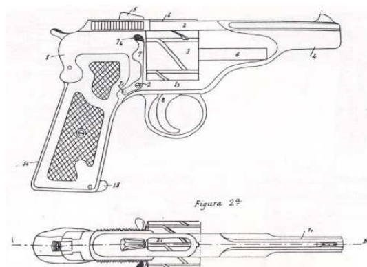
DISEÑOS DEL REVOLVER AUTOMÁTICO DE BOLSILLO, PATENTADO POR TORIBIO ZULAICA EN 1903
