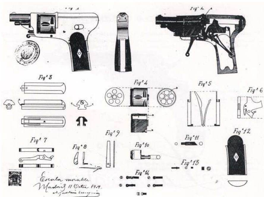
DISEÑOS DEL “REVOLVER AUTOMÁTICO DENOMINADO AGURO”, PATENTADO POR MARTÍN ERQUIAGA, EL AÑO 1909
