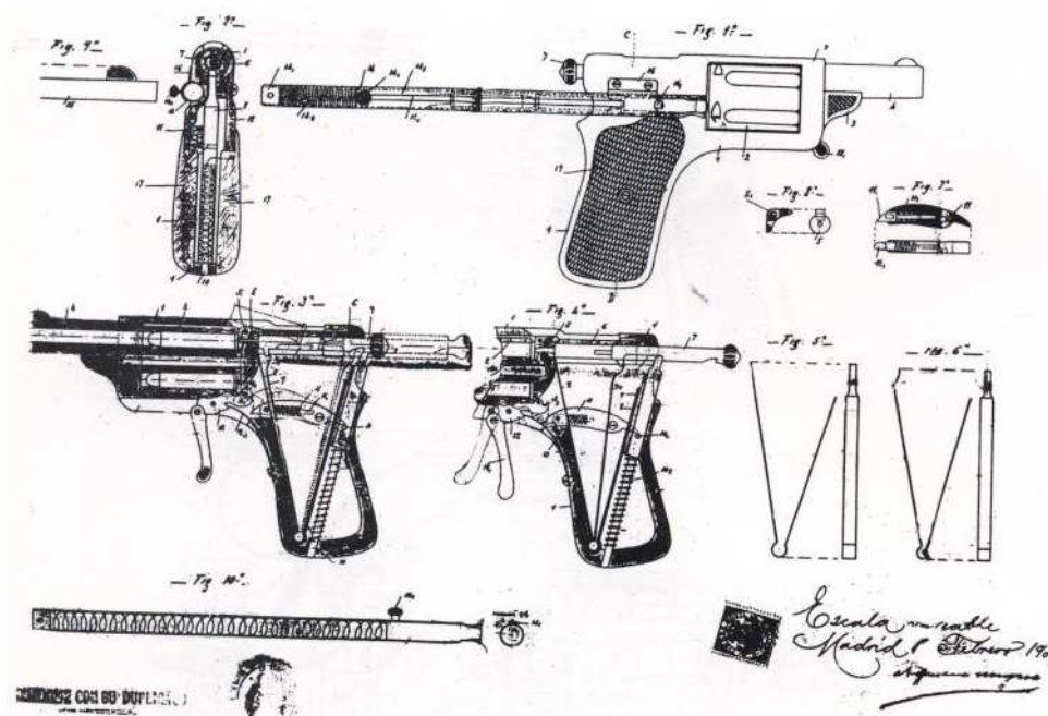
DISEÑOS DEL REVOLVER AUTOMÁTICO DE BOLSILLO, PATENTADO POR TORIBIO ZULAICA EN 1905
