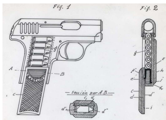
DISEÑO DE LA PISTOLA “RADIUM”, PATENTADA POR GUILLERMO ECHEVERRÍA Y VALENTIN VALLEJO, EL AÑO 1913
