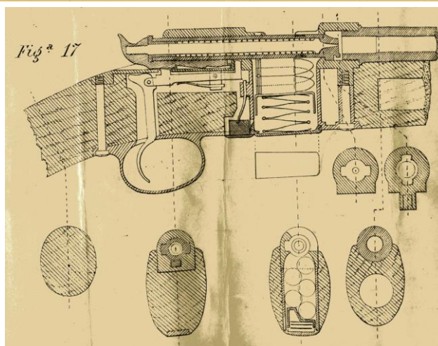
Figuras 1 y 17, ilustrando la carabina patentada en 1919 por el coronel Génova.
