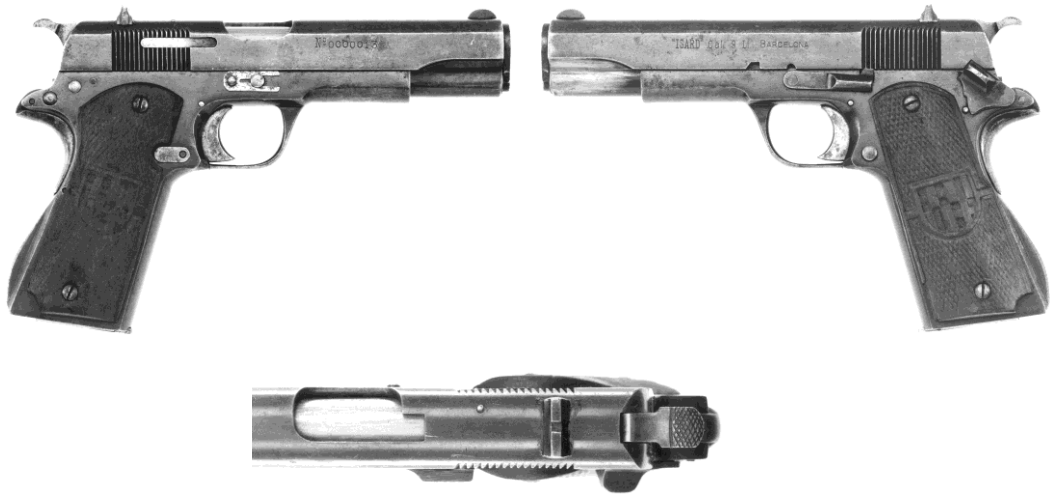
Pistola "ISARD" (Nº 13), 1º modelo, con armazón construido en única pieza y con seguro de empuñadura. (Foto Leonardo M. Antaris)
